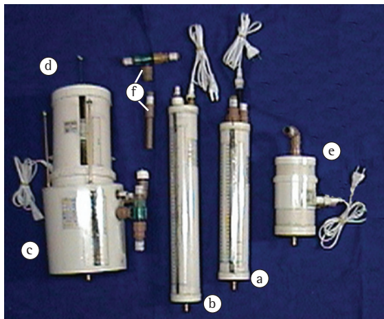
Figura 1 – Peças principais do aparelho isoladas: a) Válvula de Positive end-Expiratory Pressure (PEEP); b) Válvula de segurança; c) Cilindro principal; d) Fole; e) Umidificador; e f) Distribuidor de ar.
