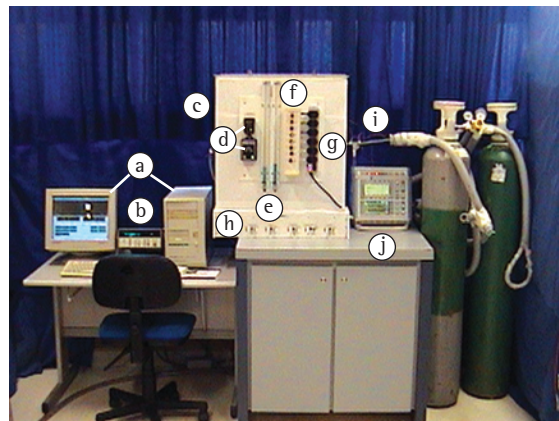
Figura 3 – Aparelho ativado sob ventilação mecânica e com coleta computadorizada de dados: a) Microcomputador com software Agilent Benchlink; b) Sistema de aquisição e controle de sinais; c) Aparelho de condicionamento; d) Termostatos do painel de controle; e) Manômetros do painel de controle; f) Chave de comando do painel de controle; g) Força elétrica do painel de controle; h) Porão; i) Cânula orotraqueal de 8 mm; e j) Ventilador mecânico.
