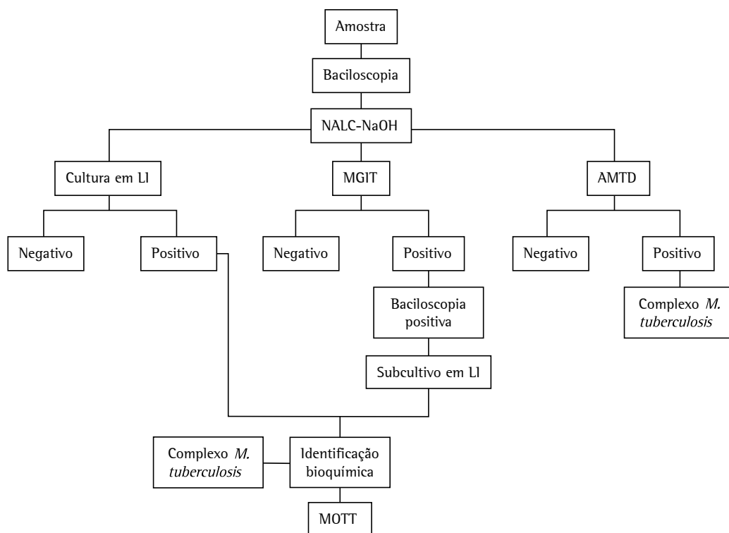
Figura 1 – Fluxo de processamento das amostras. NALC-NaOH: N-acetil-L-cisteína-hidróxido de sódio; LJ: Löwenstein-Jensen; MGIT: Mycobacteria Growth Indicator Tube ; AMTD: teste amplified Mycobacterium tuberculosis direct ; e MOTT: mycobacteria other than tuberculosis (micobactérias que não tuberculose).
